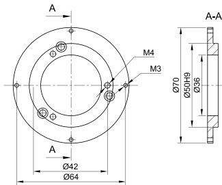
型号:9500/002 铝合金
