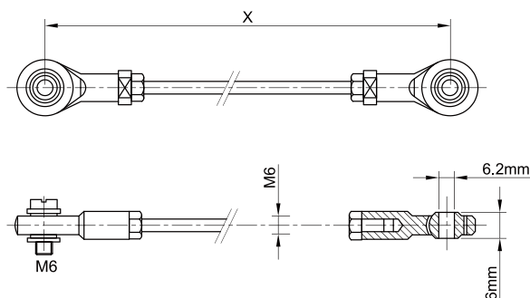
B型尺寸
