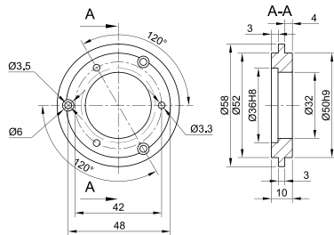
型号:9500/004 铝合金
