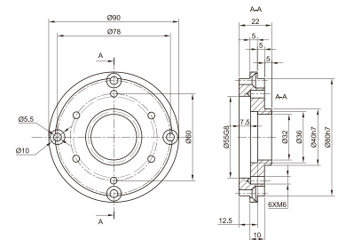
型号:9500/011 铝合金
