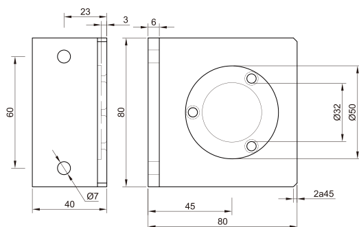
型号:9202
