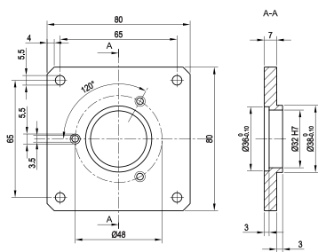
型号:9500/006 铝合金
