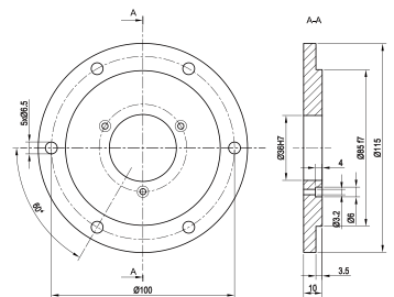
型号:9500/010 铝合金
