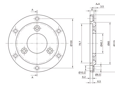
型号:9500/007 铝合金
