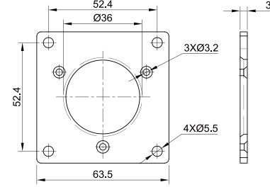
型号:9500/005 铝合金
