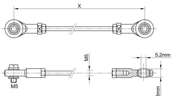
A型尺寸
